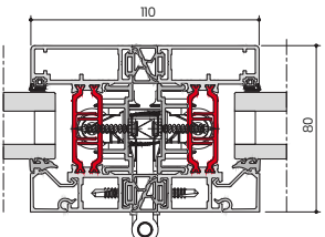
F80 COUPE HORIZONTALE OUVRANT CHARIOT
