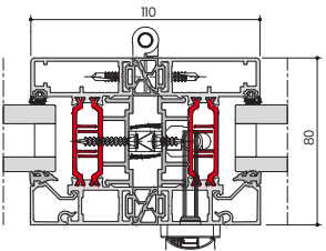
F80 COUPE HORIZONTALE VERROUILLAGE INTERMÉDIAIRE
