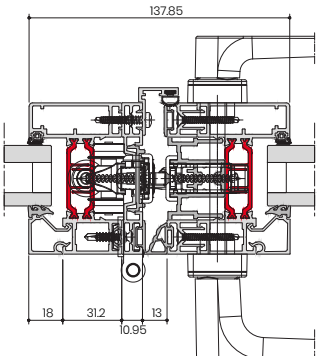
F80 COUPE HORIZ. VANTAIL DE SERVICE/ OUVRANT DEMI-CHARIOT
