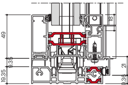
F80 COUPE VERTICALE BASSE SEUIL PMR
