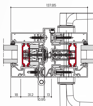
➤ F80 COUPE HORIZ. VANTAIL DE SERVICE/OUVRANT DEMI-CHARIOT
