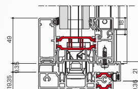
➤ F80 COUPE VERTICALE BASSE SEUIL PMR
