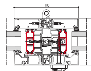
➤ F80 COUPE HORIZONTALE VERROUILLAGE INTERMEDIAIRE
