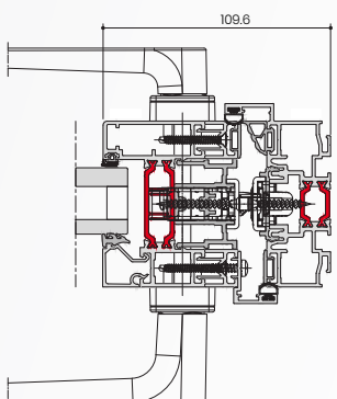
➤ F80 COUPE HORIZ. VANTAIL DE SERVICE/DORMANT
